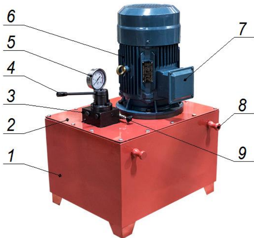
Рис.1. Устройство маслостанции
