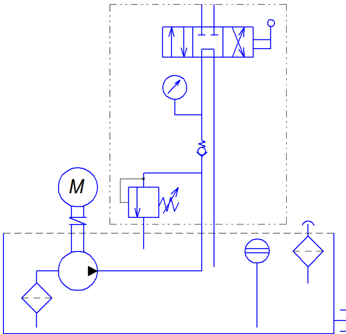
Рис.2. Гидравлическая схема МГС250-6.0-Р-2-40л-380В, МГС250-10.0-Р-2-100л-380В, МГС250-20.0-Р-2-150л-380В
