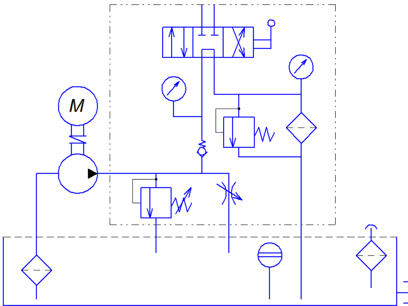
Рис.3. Гидравлическая схема МГС250-50.0-Р-2-300л-380В, МГС250-100.0-Р-2-600л-380В
